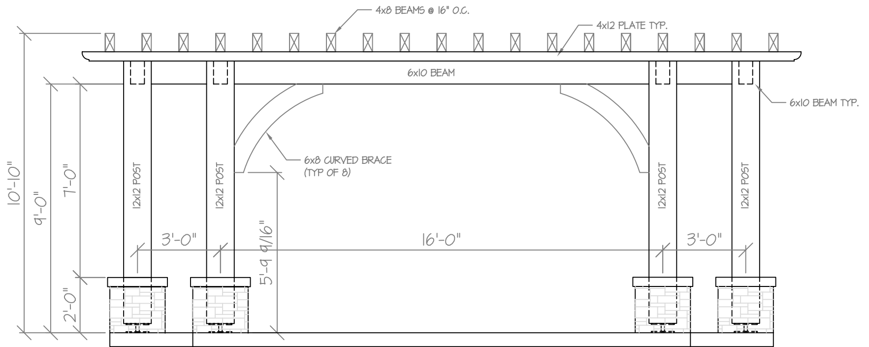
PERGOLA SECTION SCALE: 3/8"=1'-0"
