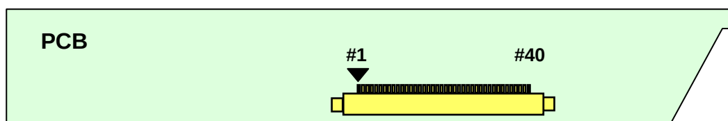
CN1 (FI-JT40S-HF10)
