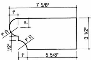
710-Cross Section
