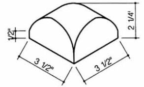
903-Coping Corner
