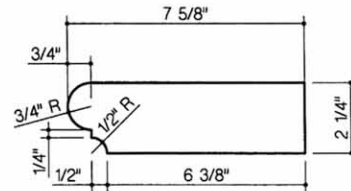
810-Cross Section
